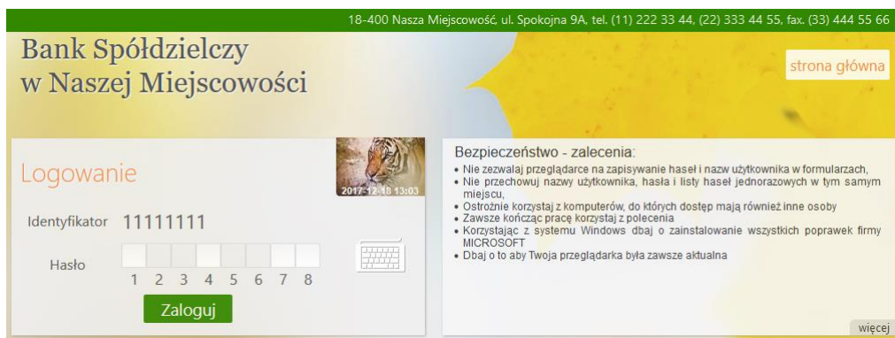
Rys.1 Okno „Logowanie”.
